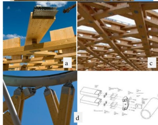
a. Lembaran plat baja sebagai pasak untuk sambungan kayu b. Sambungan kayu dengan ujung bawah atap.
