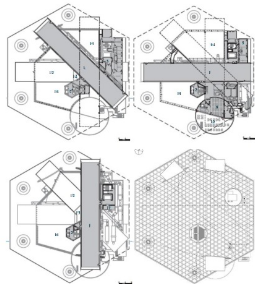
Gambar 11. Denah Lantai 2, 3, 4 dan Atap Pompidou Centre Metz
