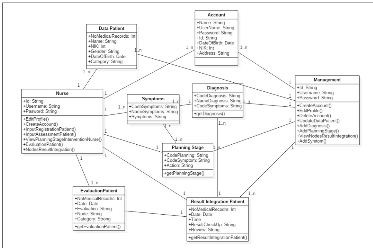
Figure 3. Class diagram MNCPIIS.
