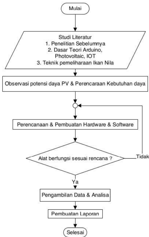
Gambar 2 Metodologi Penelitian
