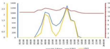
Gambar 10 Pengujian photovoltaic blok 1 cuaca Hujan
