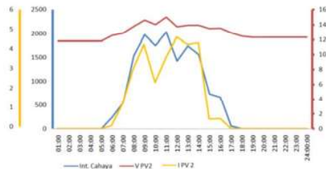
Gambar 9 Pengujian photovoltaic blok 2 cuaca cerah
