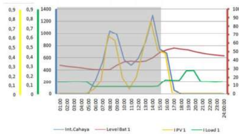
Gambar 13 Grafik performa harian sistem blok 2 pada cuaca cerah.
