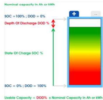
Gambar 1 Analogi SoC dan DoD baterai
