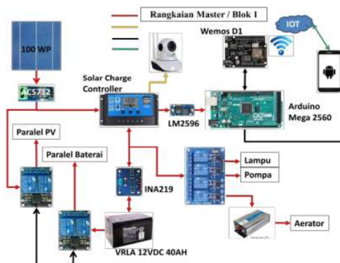
Gambar 4 Rangkaian Blok 1
