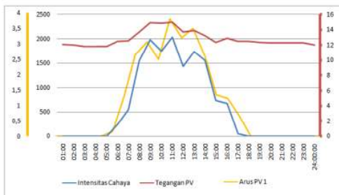
Gambar 8 Pengujian photovoltaic blok 1 cuaca cerah
