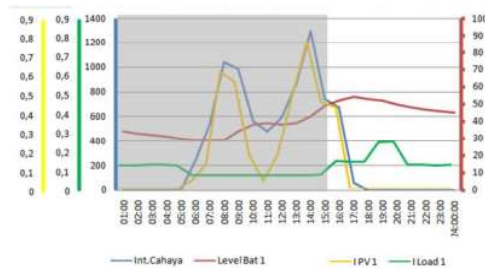
Gambar 14 Performa harian sistem blok 1 pada cuaca hujan.
