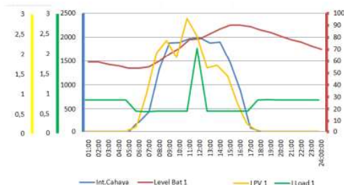
Gambar 12 Grafik performa harian sistem blok 1 pada cuaca cerah.
