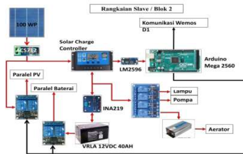
Gambar 5 Rangkaian Blok 2
