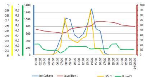
Gambar 15 Performa harian sistem blok 2 pada cuaca hujan.
