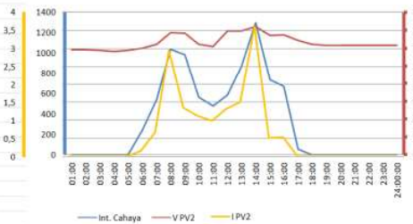
Gambar 11 Pengujian photovoltaic blok 2 cuaca hujan.
