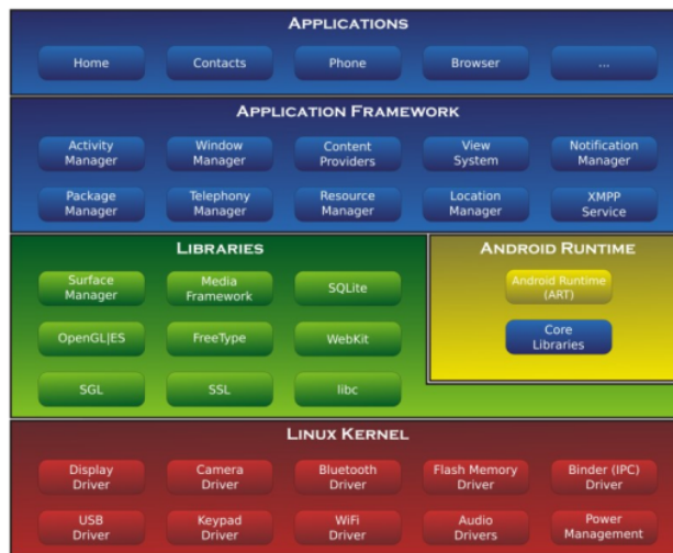
Gambar 1. Diagram Arsitektur Android
