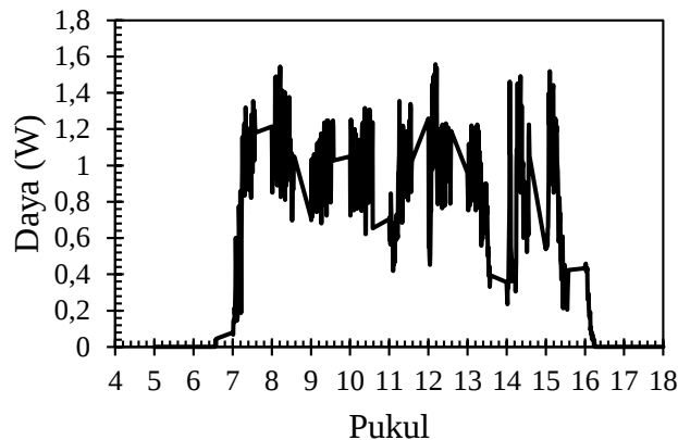
Gambar 6. Hasil pengukuran keluaran daya listrik photovoltaic cell
